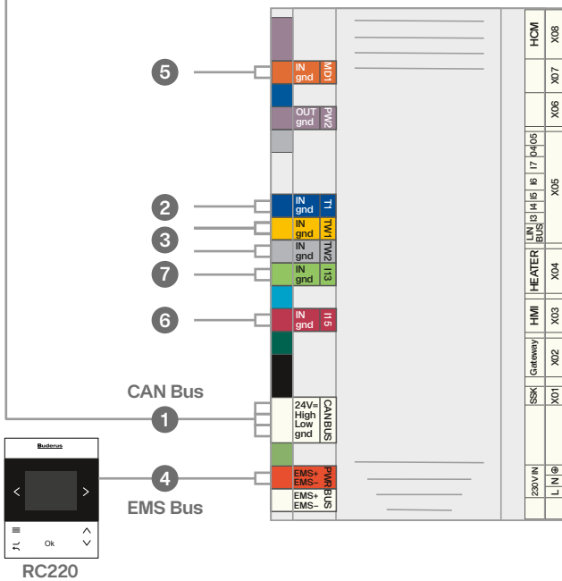
Inneneinheit Logatherm WLW186i TP70 XCU-TTH
